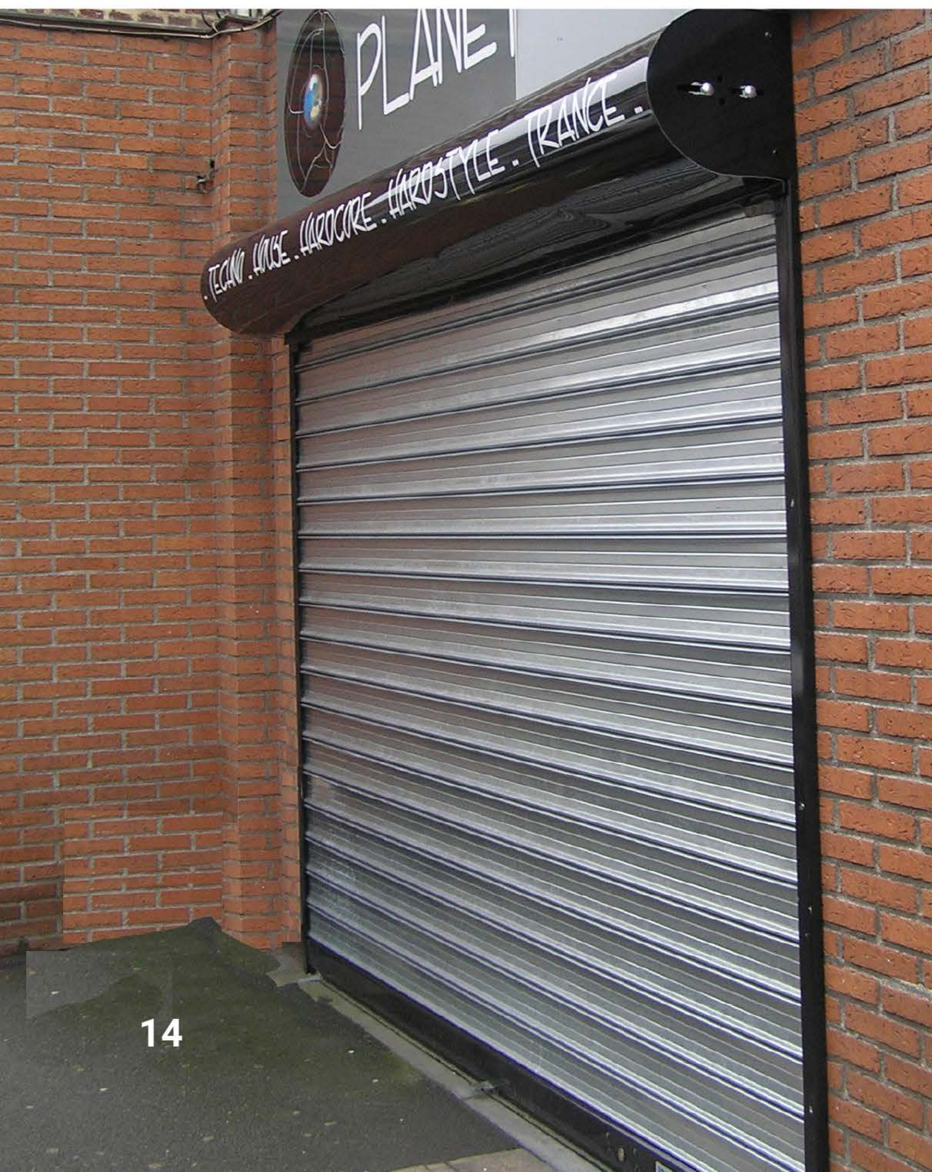
Rideau métallique 7/10ème, moteur axial. Coulisse lame finale et coffre rond laqué noir. L 3300 x H 2100 mm
